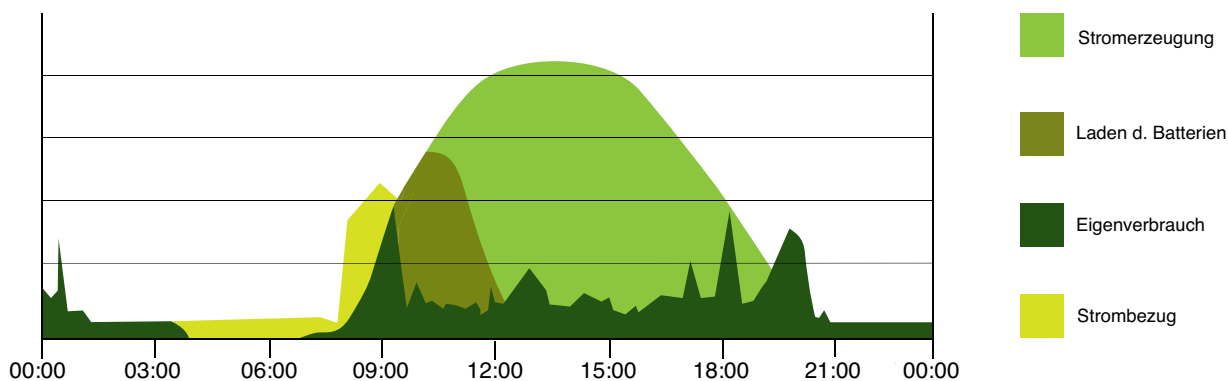
Abb. 2: Eigenverbrauchssituation mit Optimierung durch Batterien
